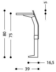
PRIMA FILA
