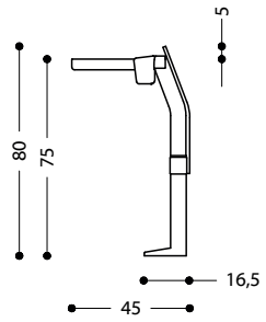
PRIMA FILA
